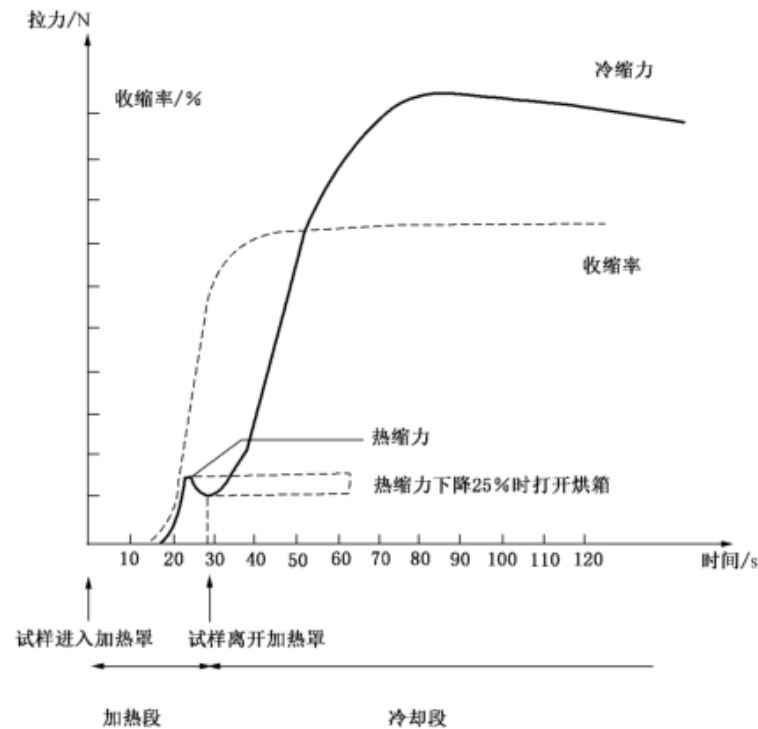
图 2 收缩力与收缩率的测定——收缩现象的典型动力学实例
