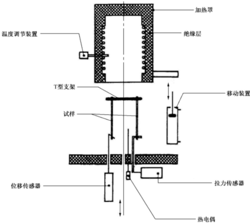
图 1 热缩仪示例图
